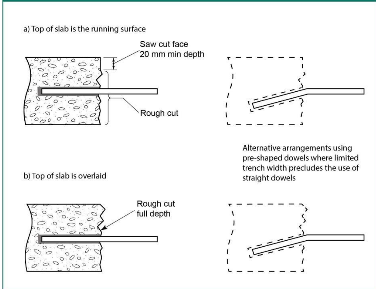
Figure S7.2 Edge options
