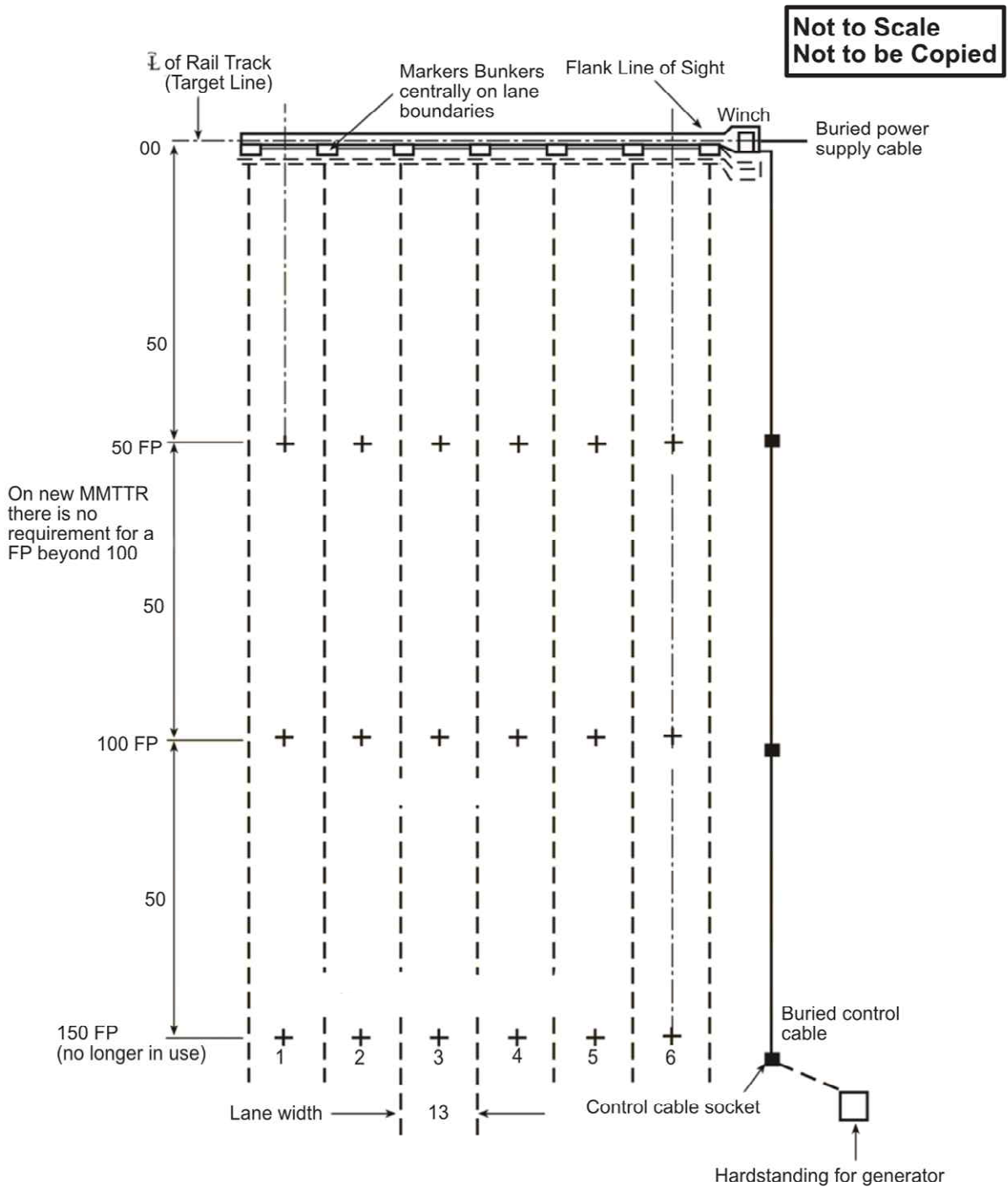
Fig 16 - 2. MMTTR Layout
