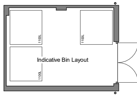
Plan 1 : 100
