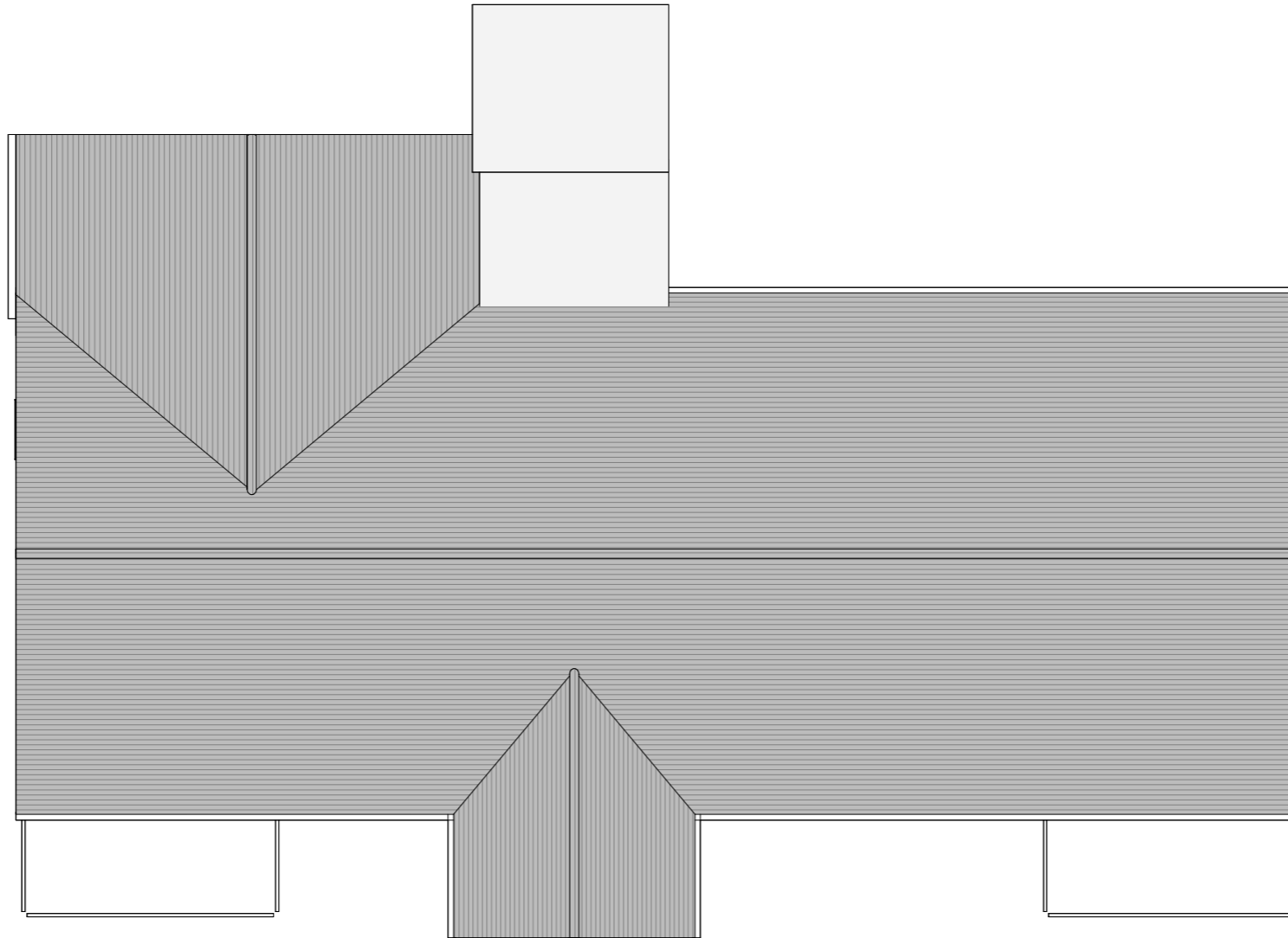
Roof Plan 1 : 100
