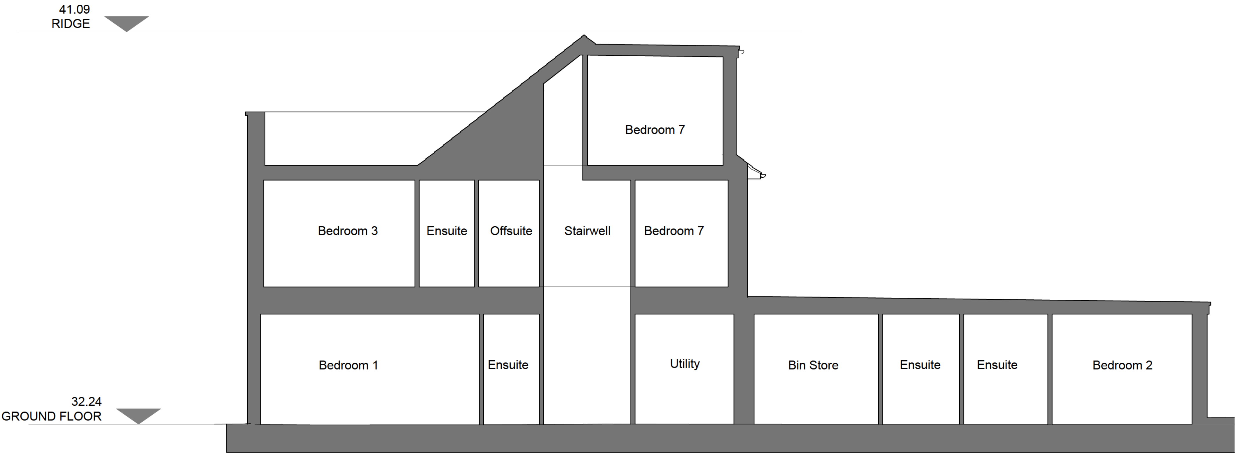
SECTION A-A
