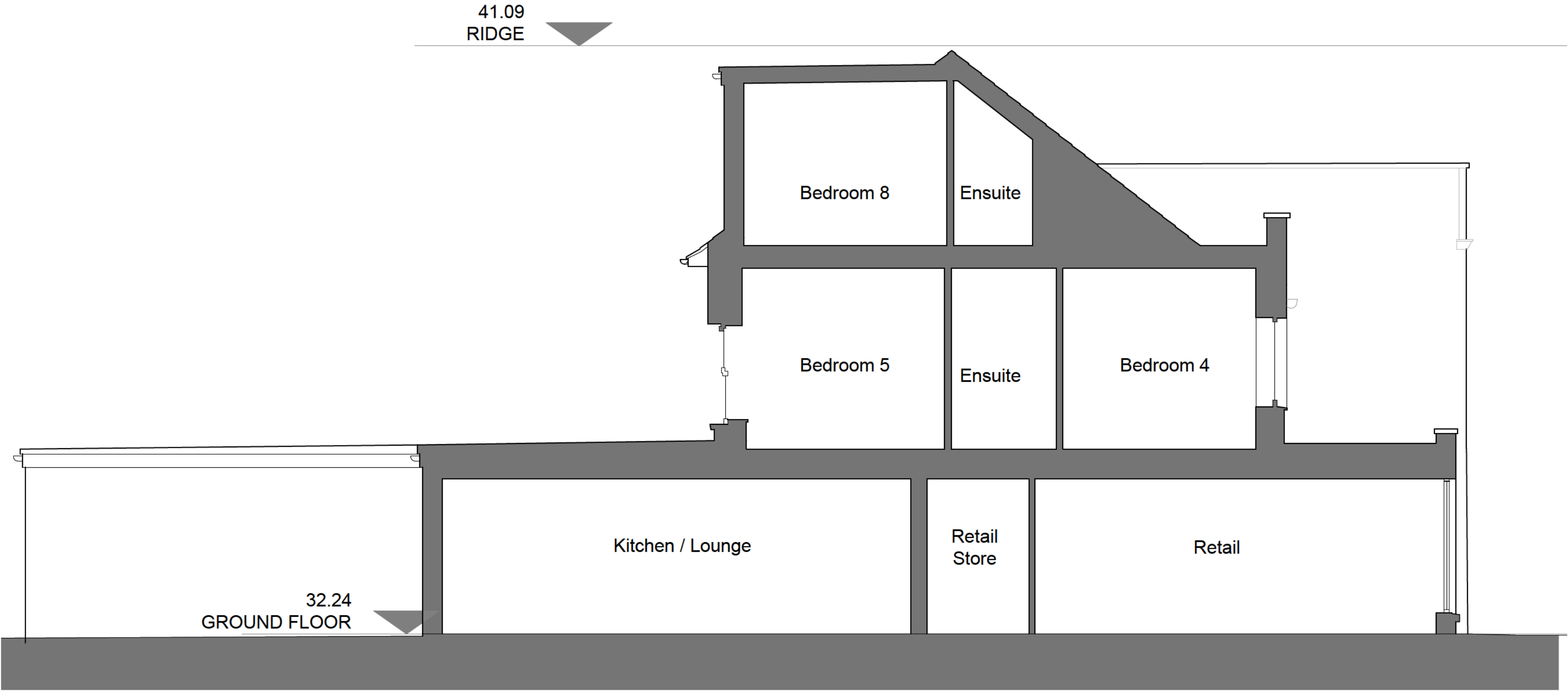
SECTION A-A
