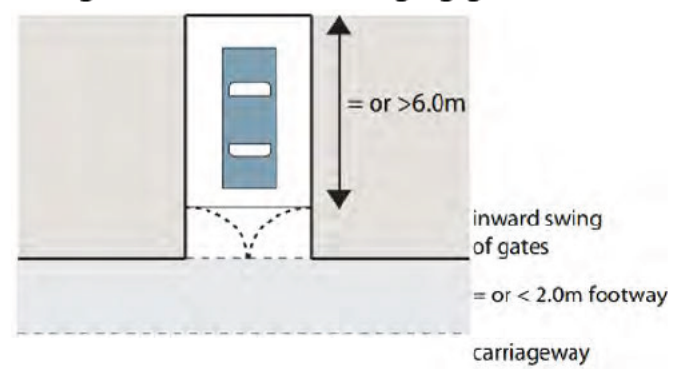
Garage Door – inward swinging gates
