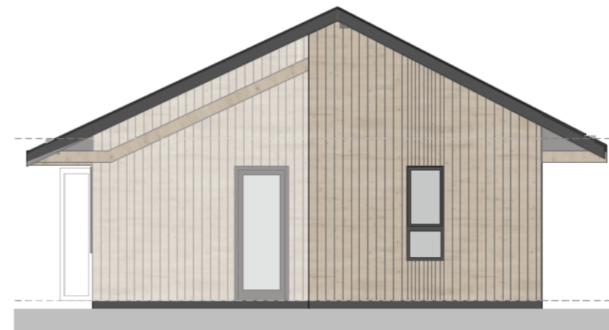
Elevation 4
