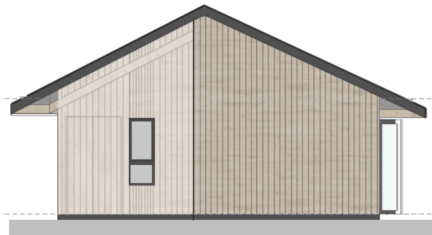
Elevation 3
