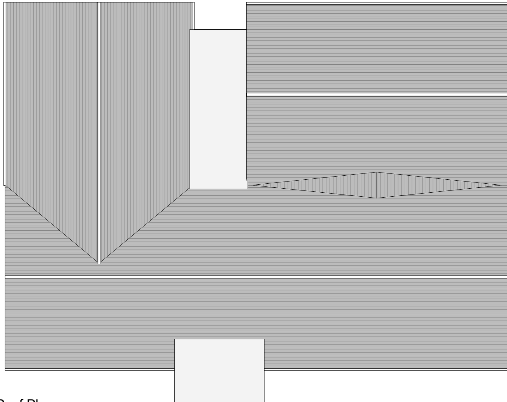
Roof Plan 1 : 100
