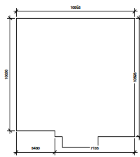
Footprint plan 1:100
