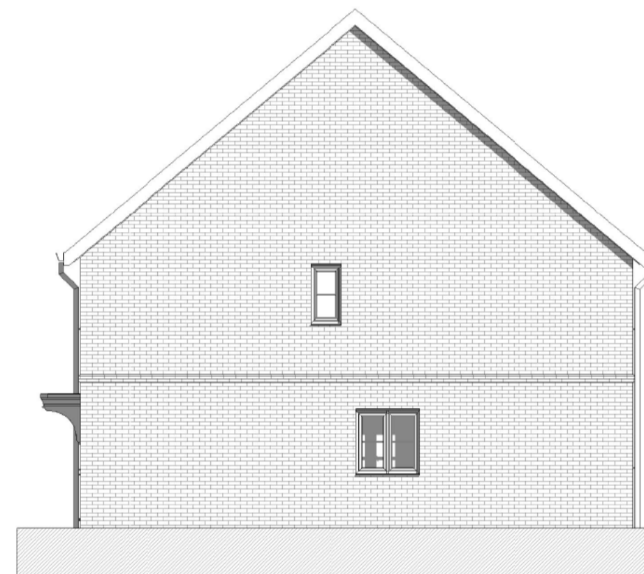
Right elevation 1 : 100
