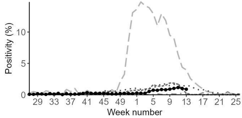
Influenza B
