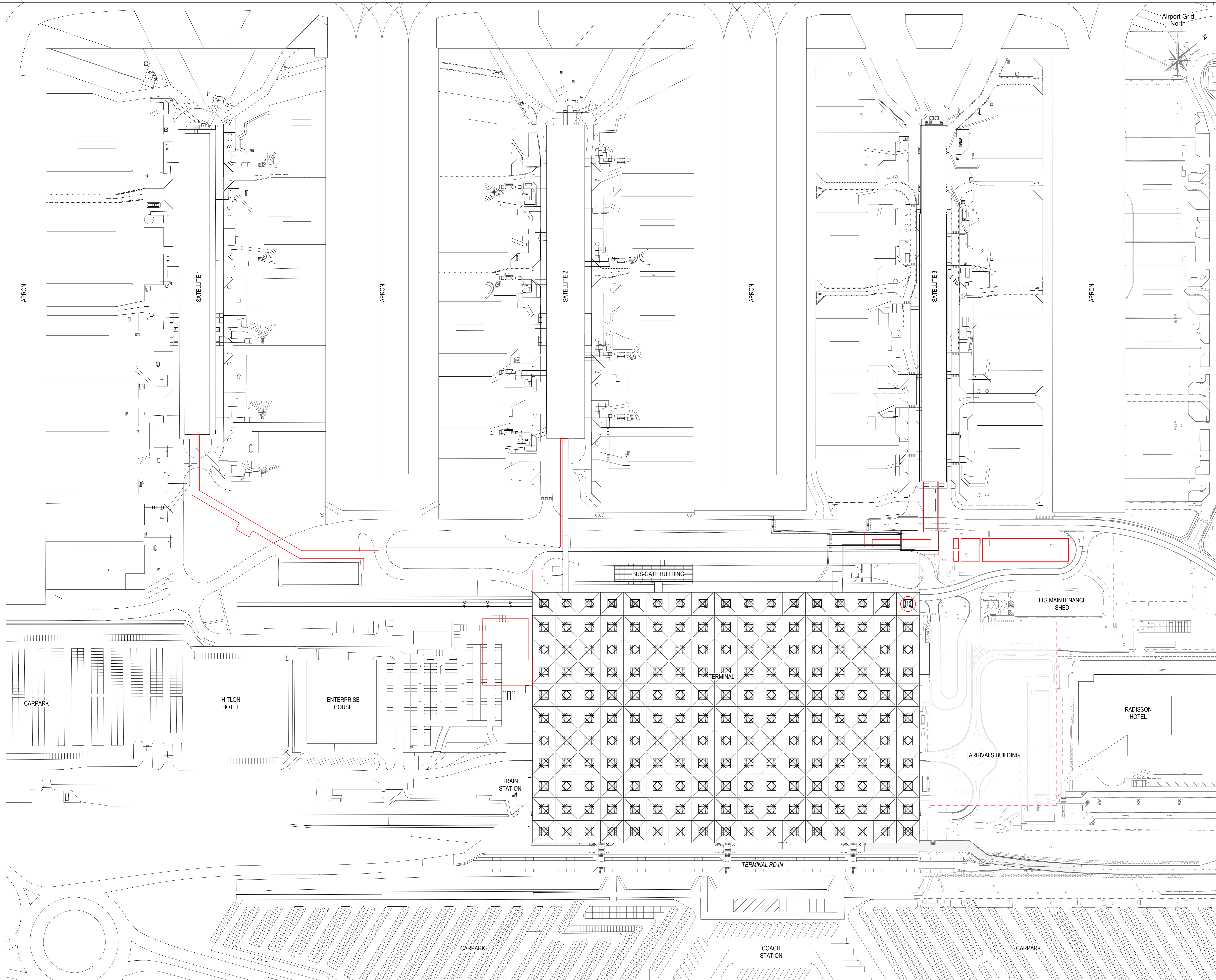
1 STN.TL- SITE PLAN - EXISTING 1:1000
