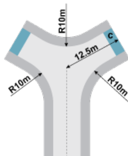
Size 2, Y Turn
