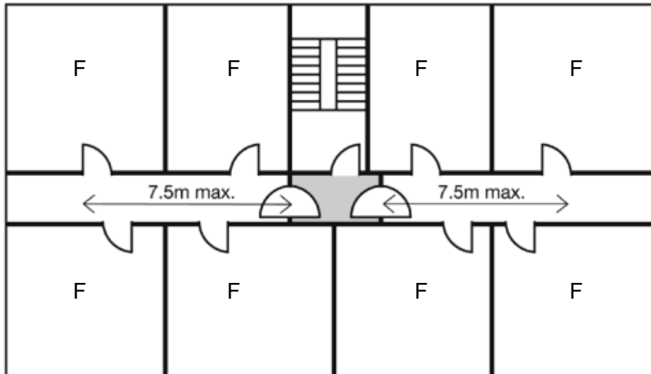
A. Corridor access flats
