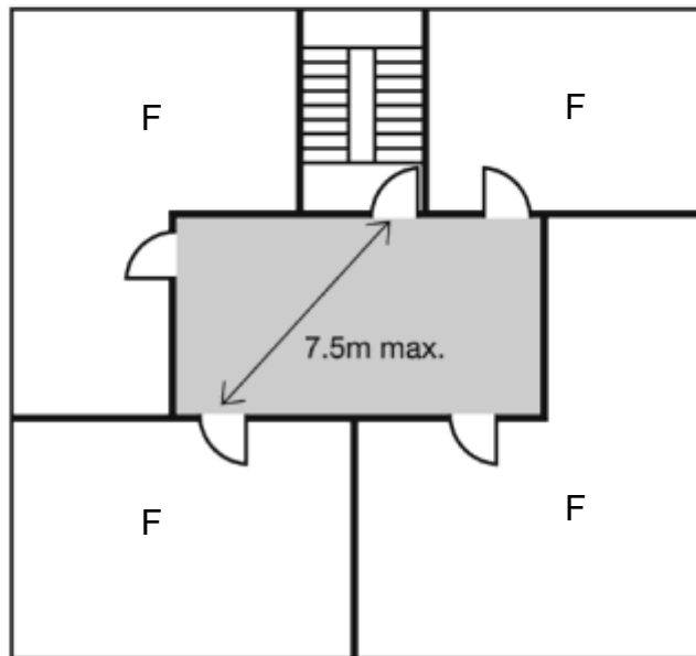
B. Lobby access flats
