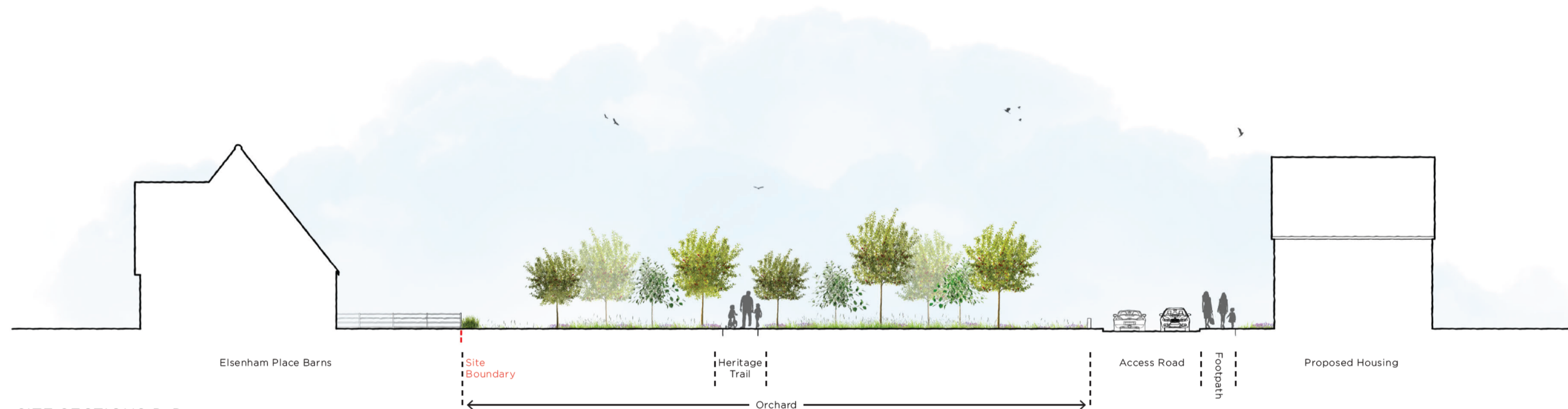
SITE SECTIONS D-D
