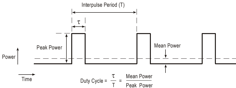
11-2 Fig 2 Pulse Radar Parameters
