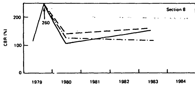
FIGURES 9a-9c In situ CBR values of the concrete bases.
