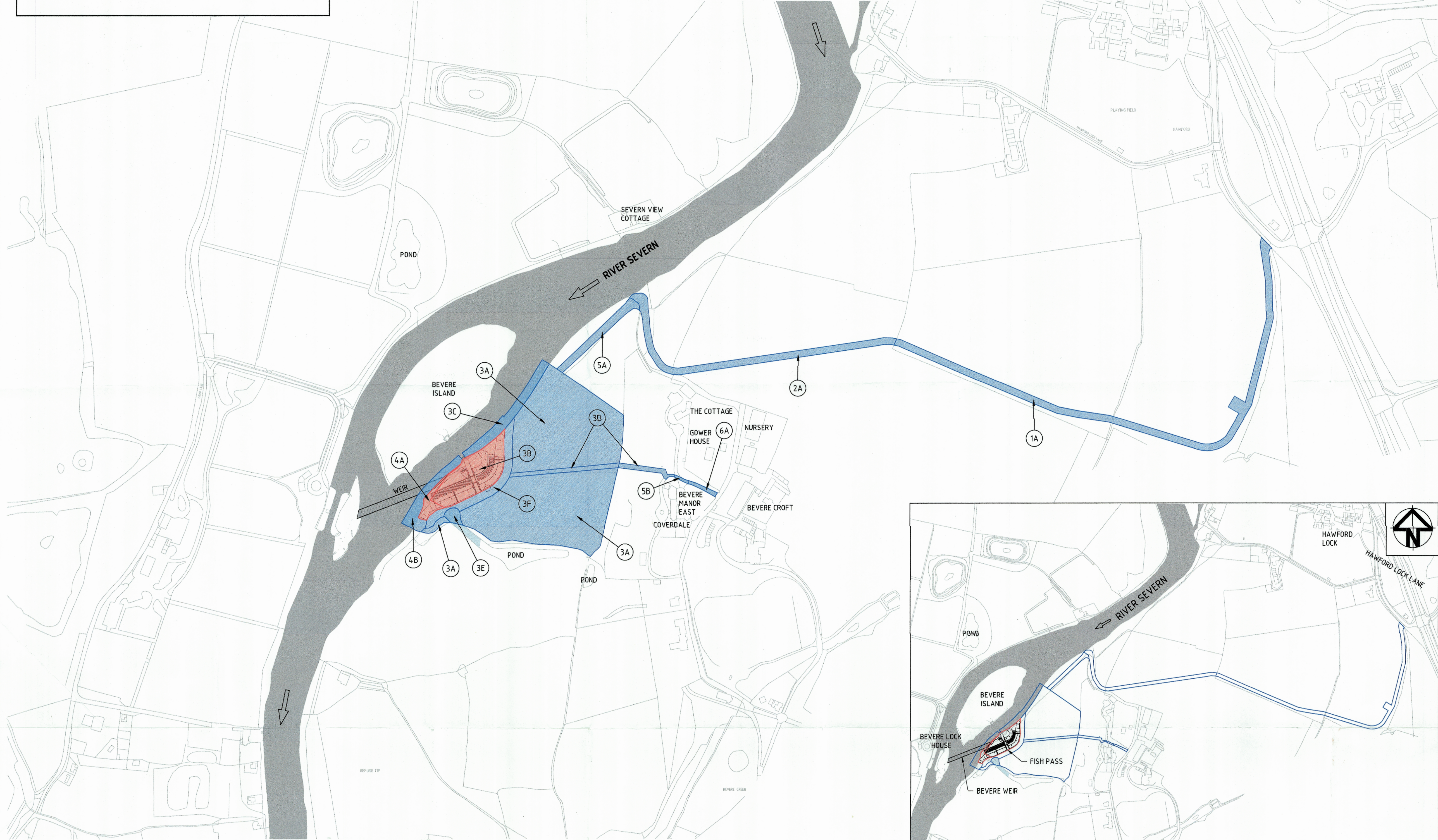
PLAN 1:2500
