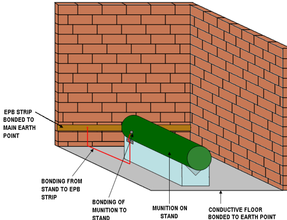
Fig 2 Equipotential Bonding of Munitions
