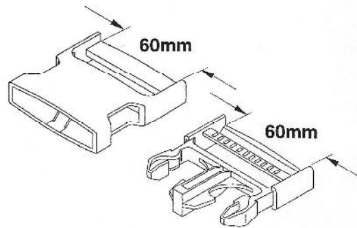
SR 60 NSN 8315-99-464-6606
