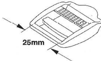
LL25 NSN 8315-99-430-3259
