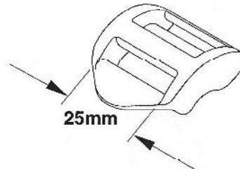
SLL25 NSN 8315-711-6724
