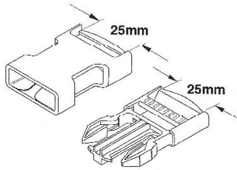
SR 25 NSN 8315-99-656-4968
