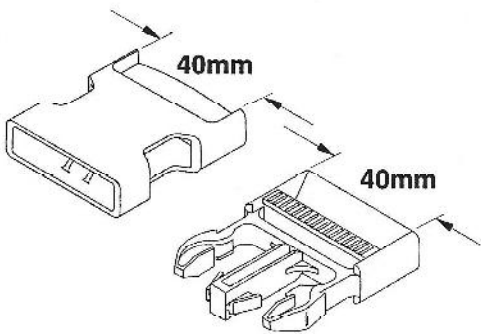
SR 40 NSN 8315-99-168-5536
