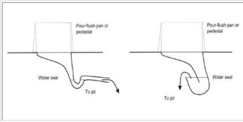
Figure 3: Varieties of pour flush latrines
