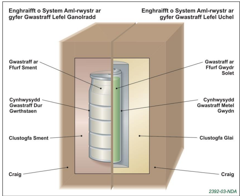
Diagram o enghraifft o systemau aml-rwystr
